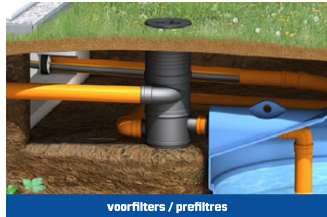
voorfilters / prefiltres
